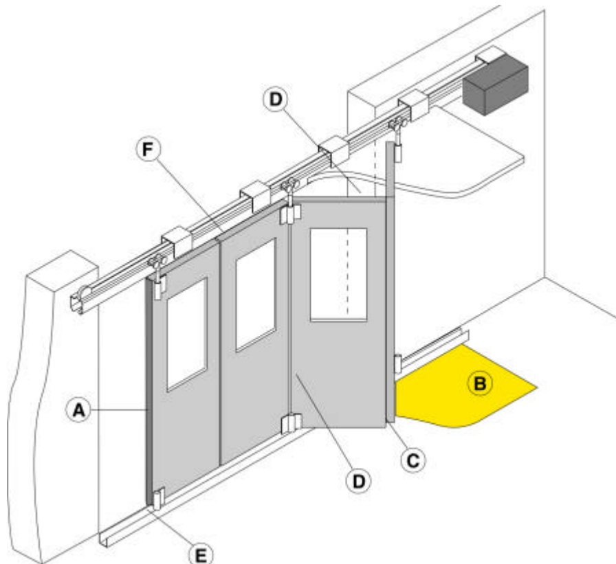
Zona de riesgos de la puerta a libro (figura 1)
